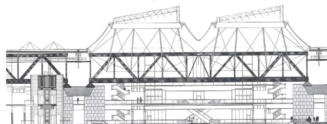
COUPE LONGITUDINALE
