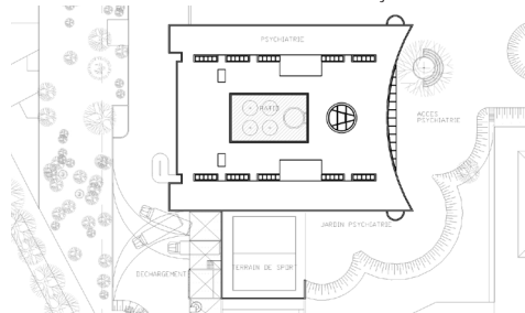
PLAN DE MASSE
