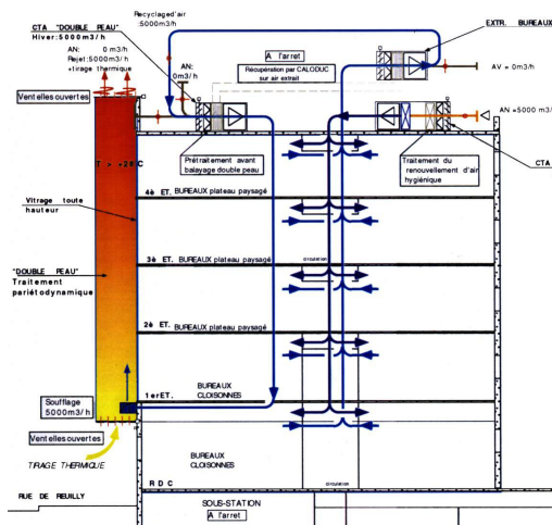
FONCTIONNEMENT DE LA FACADE BIOCLIMATIQUE
